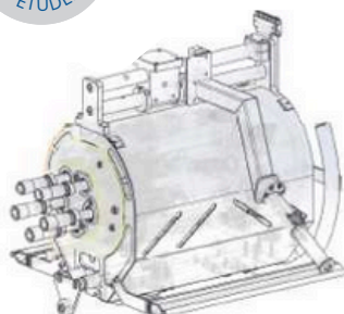
Visseuse de roues voitures multibroche à double entraxe
